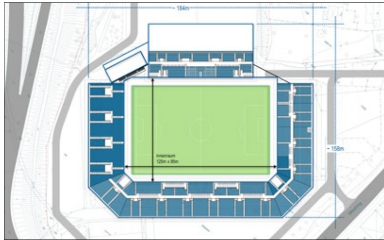
Einer von mehreren Planungsansätzen aus der Markterkundung vom Sommer 2024. Die Planungen dienen als Bemessungsgrundlagen. Der aktuell gestartete Wettbewerb wird am Ende entscheiden, wie und in welcher Form gebaut wird. Grafik: AS+P
