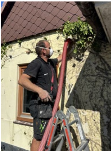
Durch den Schlauch wird feinfaserige Glaswolle in die Luftschicht des zweischaligen Mauerwerks geblasen.
